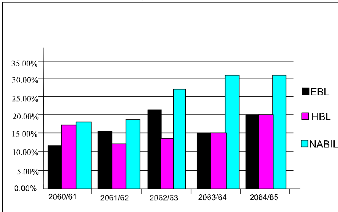
ROCE of EBL, HBL and NABIL Banks
